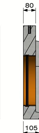
Sectie A-A (Schaal 1 : 15)
