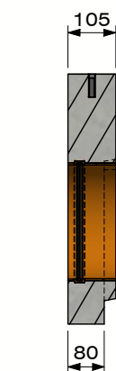
Sectie A-A (Schaal 1 : 15)
