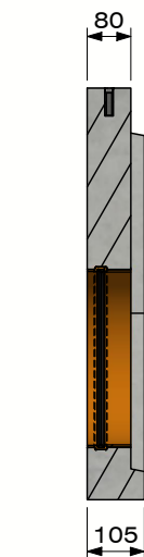
Sectie A-A (Schaal 1 : 15)
