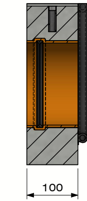
Section A-A (Echelle 1 : 7.5)
