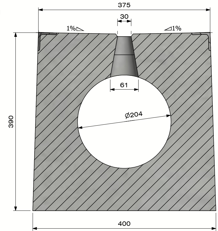
Section B-B (Echelle 1 : 5)
