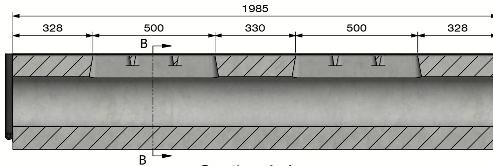
Section A-A (Echelle 1 : 15)
