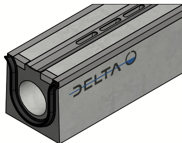
Liaison pression par joint EPDM
