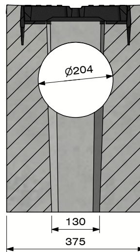
Section A-A (Echelle 1 : 10)
