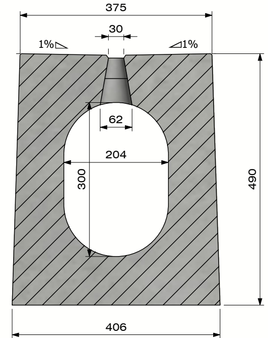
Section B-B (Echelle 1 : 7,5)
