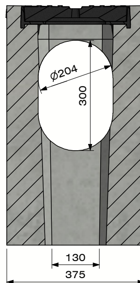
Section A-A (Echelle 1 : 10)
