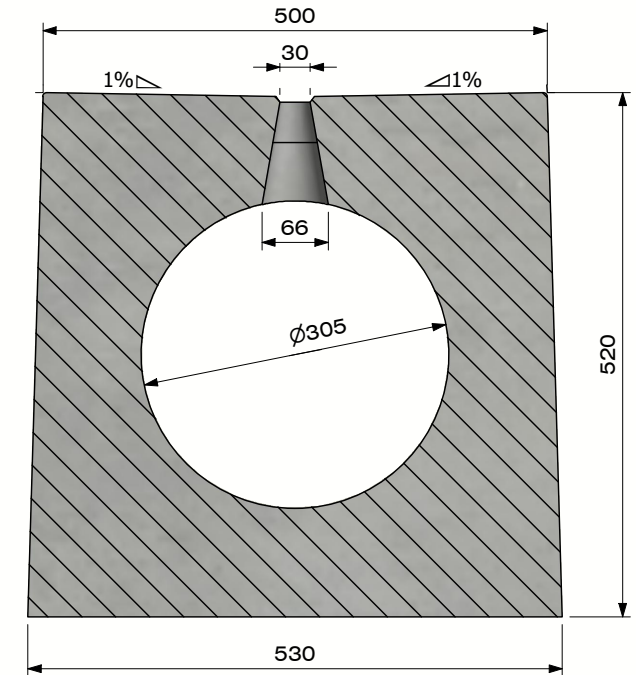
Section B-B (Echelle 1 : 7.5)
