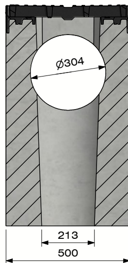
Section A-A (Echelle 1 : 15)
