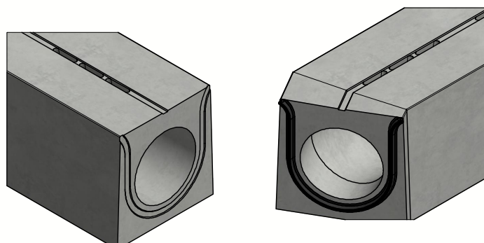
Liaison pression par joint EPDM
