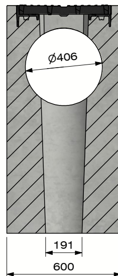
Section A-A (Echelle 1 : 20)
