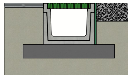
Principe type I (Consulter les prescriptions de pose)
