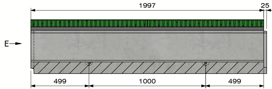
Section D-D (Echelle 1 : 20)
