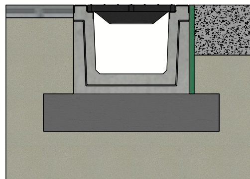
Principe type I (Consulter les prescriptions de pose)
