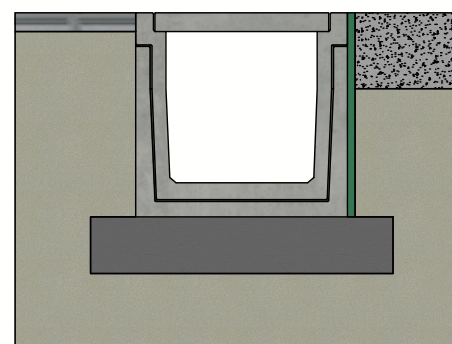
Principe type I (Consulter les prescriptions de pose)
