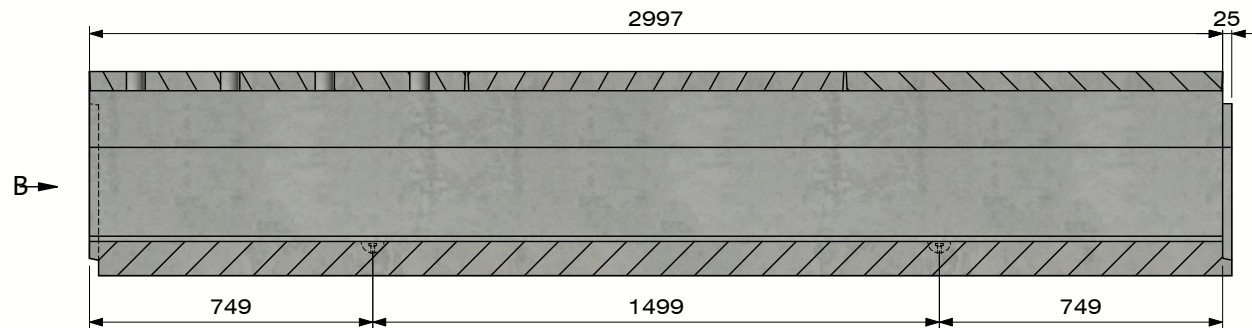
Section A-A (Échelle 1 : 20)
