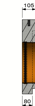
Section A-A (Échelle 1 : 15)
