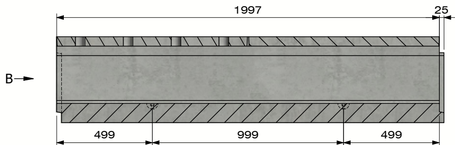
Section A-A (Échelle 1 : 20)
