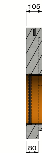
Section A-A (Échelle 1 : 15)
