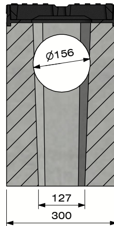
Sectie A-A (Schaal 1 : 10 )
