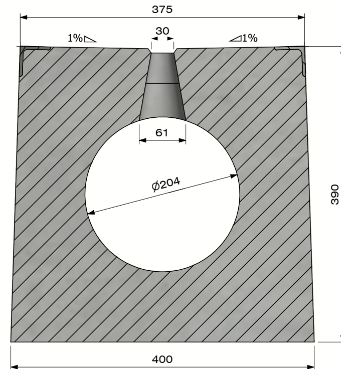
Sectie B-B (Schaal 1 : 5)
