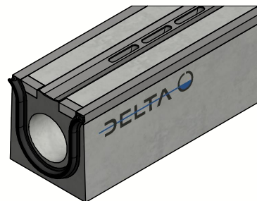
Drukverbinding met EPDM rubberdichting
