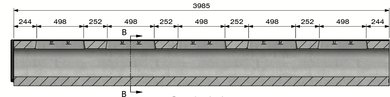
Sectie A-A (Schaal 1 : 25)
