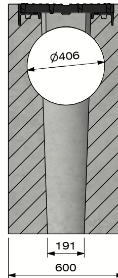
Sectie A-A (Schaal 1 : 20)
