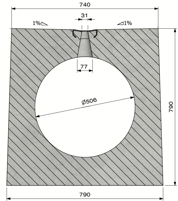
Section B-B (Echelle 1 : 10)
