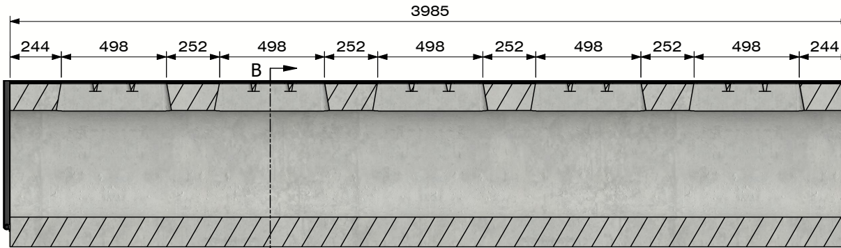
Section A-A (Echelle 1 : 25)
