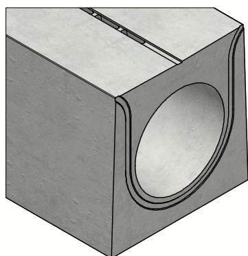
Drukverbinding met EPDM rubberdichting
