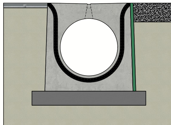
Principe type I (Raadpleeg de plaatsingsvoorschriften)
