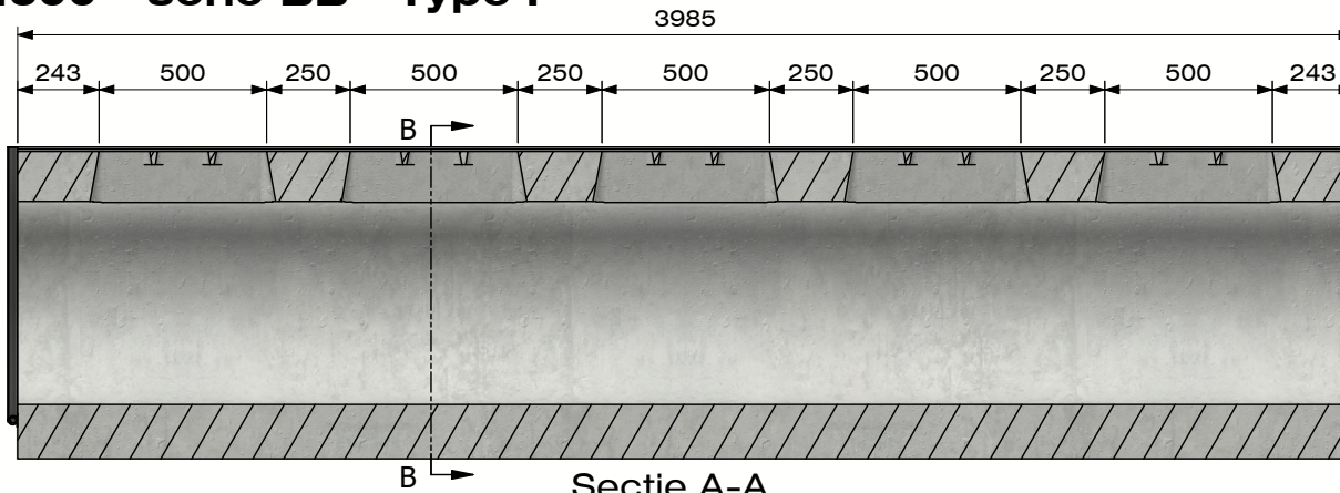
Sectie A-A (Schaal 1 : 25)
