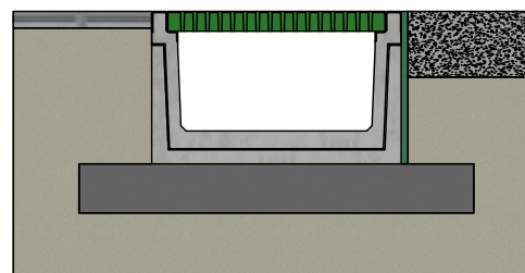
Principe type I (Raadpleeg de plaatsingsvoorschriften)
