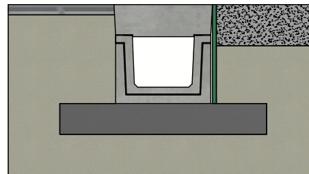
Principe type I (Raadpleeg de plaatsingsvoorshriften)
