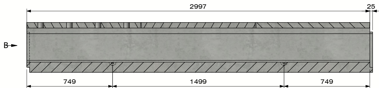
Sectie A-A (Schaal 1 : 20)
