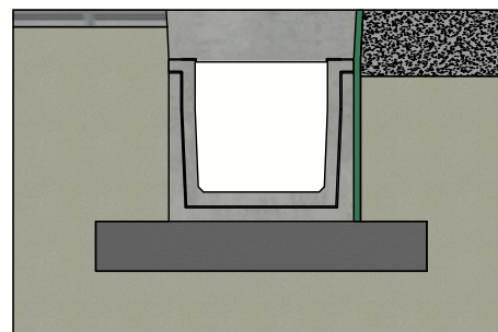
Principe type I (Raadpleeg de plaatsingsvoorshriften)
