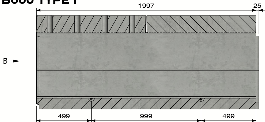
Sectie A-A (Schaal 1 : 20)
