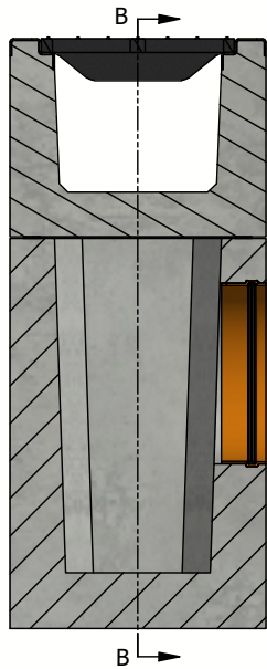
Sectie : A-A (Schaal : 1 : 15)
