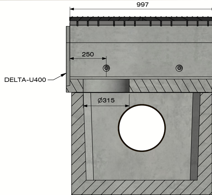
Sectie : D-D (Schaal : 1 : 15)
