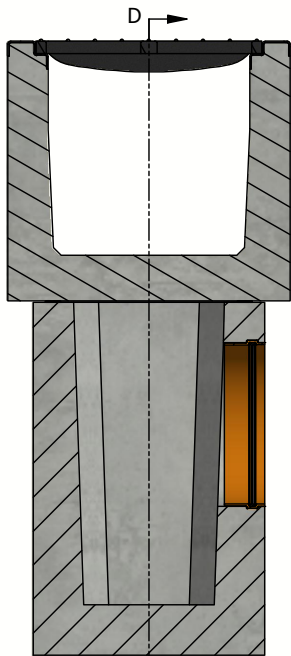
Sectie : C-C (Schaal : 1 : 15)
