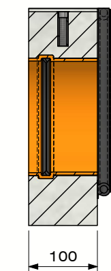
Sectie A-A (Schaal 1 : 7.5)
