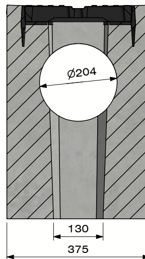
Sectie A-A (Schaal 1 : 10)
