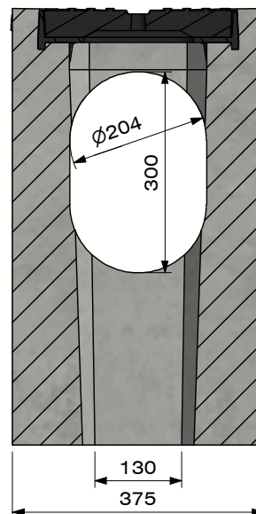
Sectie A-A (Schaal 1 : 10 )
