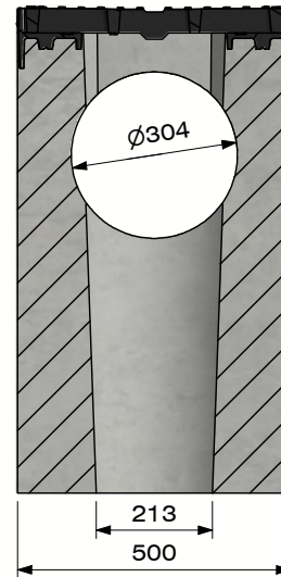
Sectie A-A (Schaal 1 : 15)
